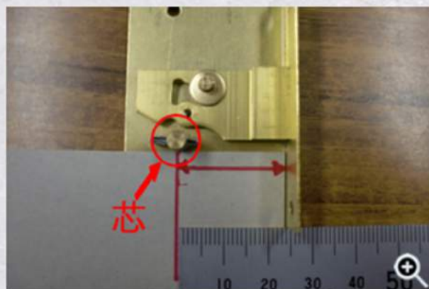
③ 芯の形状を確認
