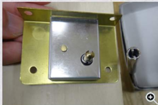
② 両溝錠(両溝鍵が対応)
