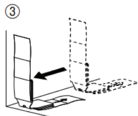
○ 取付図
