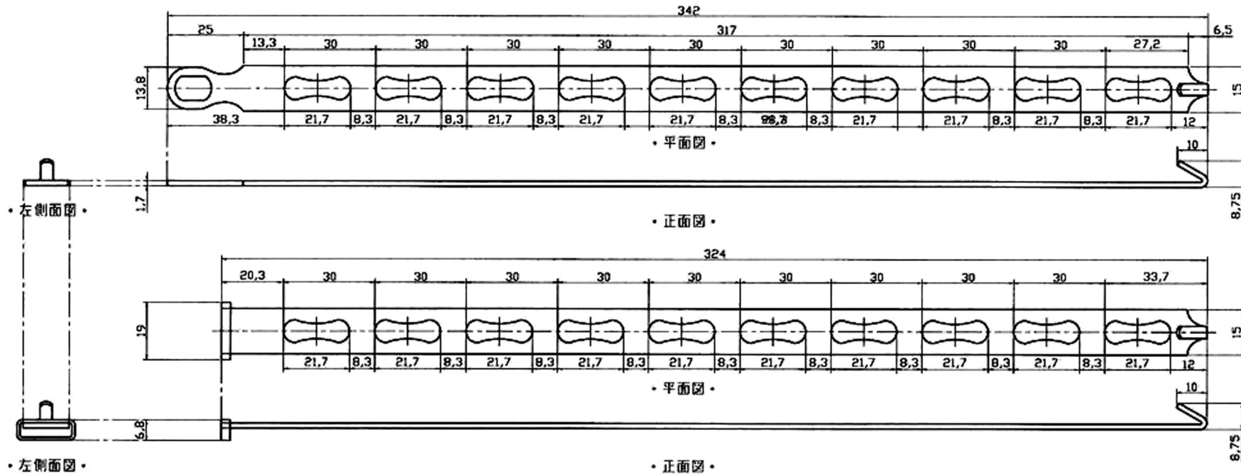
＜兵丹自在吊り 本体図＞
