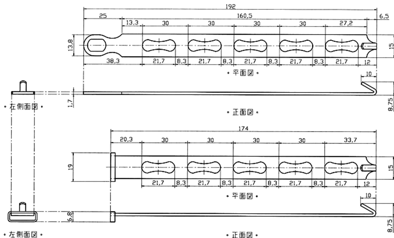
＜兵丹自在吊り 本体図＞ S=1:1
