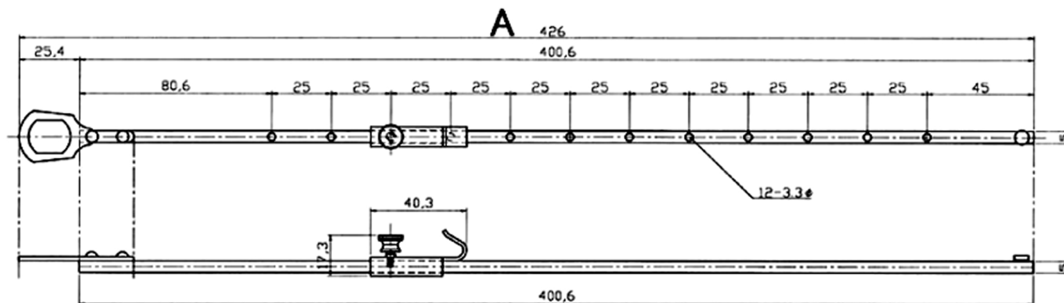
<角線自在吊 全体図/S=1:1.5>
