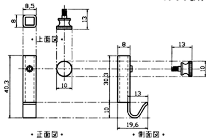
<フック部分 詳細図/S=1:1>
