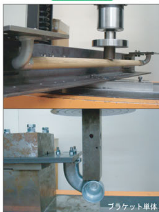
水平荷重試験
