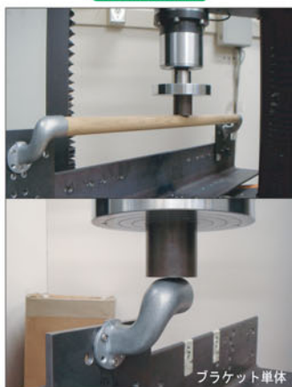
垂直荷重試験
