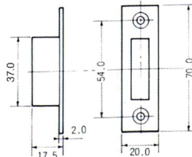
掘込受座 B
