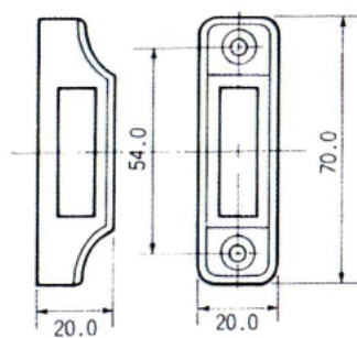
共通受座 A
