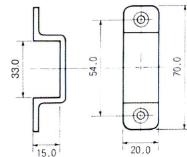
ロングラッチ用中間座
