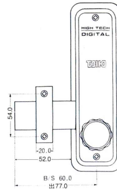
ロングラッチタイプ
