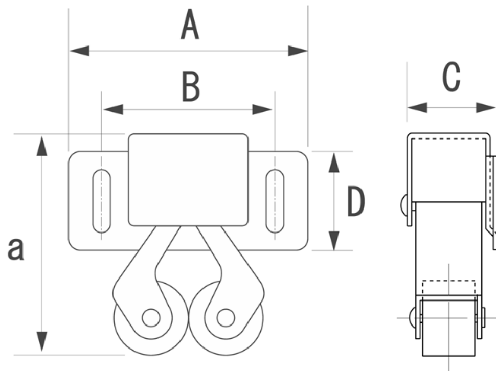
本体
