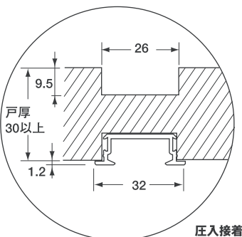
圧入接着
